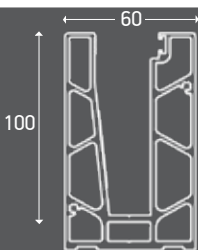
SD-6030 | 2,35kg ΟΡΙΖΟΝΤΙΑ ΔΙΑΤΡΗΤΗ ΤΡΑΒΕΡΣΑ Horizontal Perforated Transom Ø30
