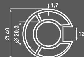
SD-5005B | 4,90kg ΣΩΛΗΝΑ Ø40 Ø40 Tube
