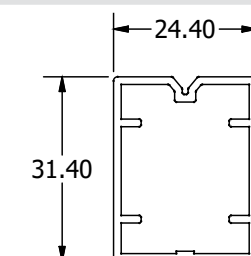
7003EX | 4.40 Kg/m Προφίλ γεμίσματος οριζόντιο Decorative Profile 32x25mm
