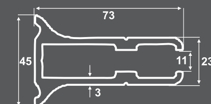
SD-6011 | 11,50kg ΠΡΟΦΙΛ ΔΑΠΕΔΟΥ ΤΖΑΜΙΟΥ 73x45mm On floor profile for glass 73x45mm
