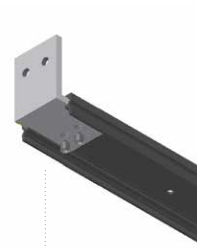
Ένωση γωνίας με οδηγό Corner joint with guide
