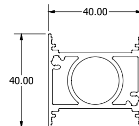
405 | 10.12 Kg/m Κολώνα 40 x 40 Column 40 x 40
