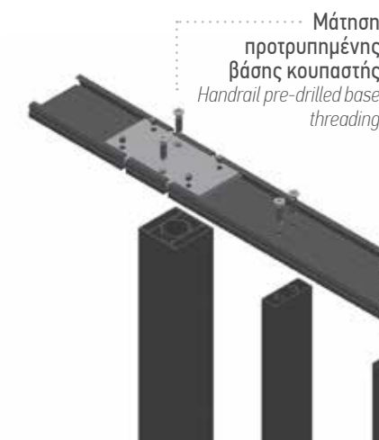
Ένωση προφίλ γεμίσματος με διάτρητη βάση κουπαστής Filler profile to Perforated Handrail Base connection
