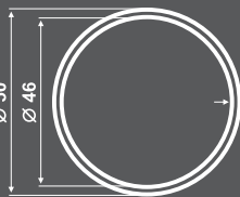
SD-5004 | 0,40kg ΚΑΠΑΚΙ ΚΟΛΩΝΑΣ ΓΙΑ 5005 & 5005A Cover for 5005 & 5005A
