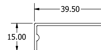
404L | 2.53 Kg/m Καπάκι διάτρητου οδηγού Perforated guide cover
