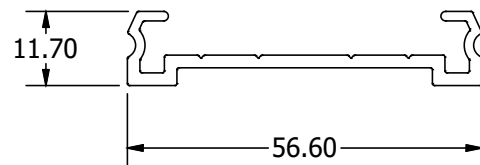
400H | 4.57 Kg/m Βάση κουπαστής Handrail base
