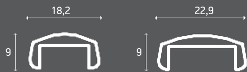
SD-6012S ΠΡΟΦΙΛ ΤΖΑΜΙΟΥ 12mm Glass profile 12mm
