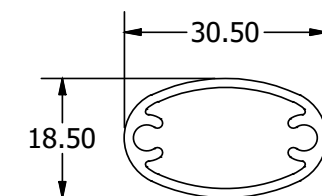
406C | 3.70 Kg/m Προφίλ γεμίσματος Filler Profile
