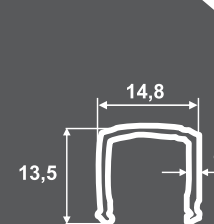
SD-6015 | 0,70kg ΚΑΠΑΚΙ ΚΟΛΩΝΑΣ ΤΖΑΜΙΟΥ Glass Column Cover
