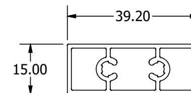
406L | 4.89 Kg/m Προφίλ γεμίσματος Filler Profile
