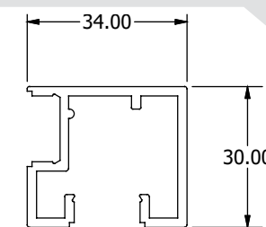
7003 | 3.70 Kg/m Οδηγός με κανάλι Transom with groove
