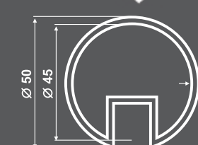
SD-6012 | 6,00kg ΚΟΥΠΑΣΤΗ ΤΖΑΜΙΟΥ Ø50 Handrail glass Ø50
