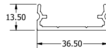
403L | 3.00 Kg/m Διάτρητος οδηγός Perforate guide
