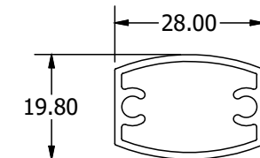
406A | 3.68 Kg/m Προφίλ γεμίσματος Filler Profile
