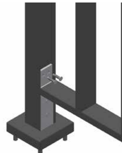
Ένωση οδηγού με κολώνα Perforated Guide to Column connection
