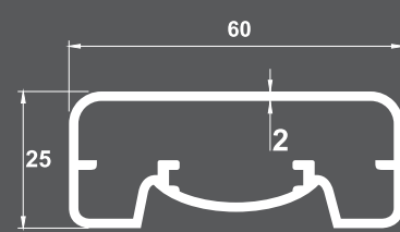
SD-6200 | 6,00kg ΚΟΥΠΑΣΤΗ 25X60mm Handrail 25x60mm
