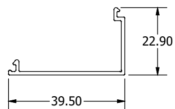
404D | 2.21 Kg/m Καπάκι διάτρητου οδηγού Perforated guide cover
