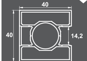
SD-7005N | 6,30kg ΚΟΛΩΝΑ 40X40mm Column 40x40mm
