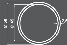
SD-5000N | 4,45kg ΚΟΥΠΑΣΤΗ Ø50 - ΕΛΑΦΡΙΑ Handrail Ø50 - Light
