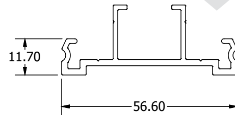
400D | 6.12 Kg/m Διάτρητη βάση κουπαστής Perforated handrail base
