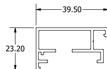
403D | 4.70 Kg/m Διάτρητος οδηγός Perforated Guide
